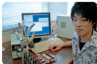
ワイヤ駆動方式多指ロボットハンド
